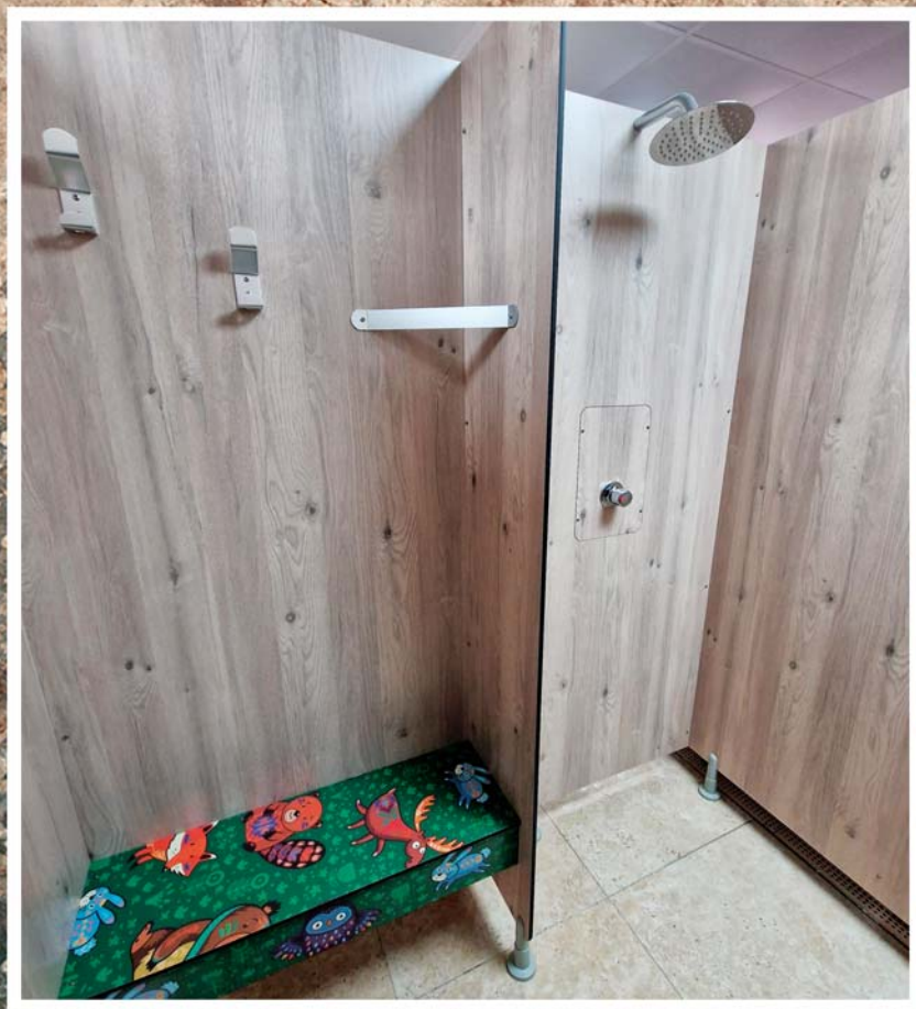
DOUCHE EN ANGLE ACZ/F51 ou ACZ/F52 355 x 1275mm ou 355 x 1928/2000mm
